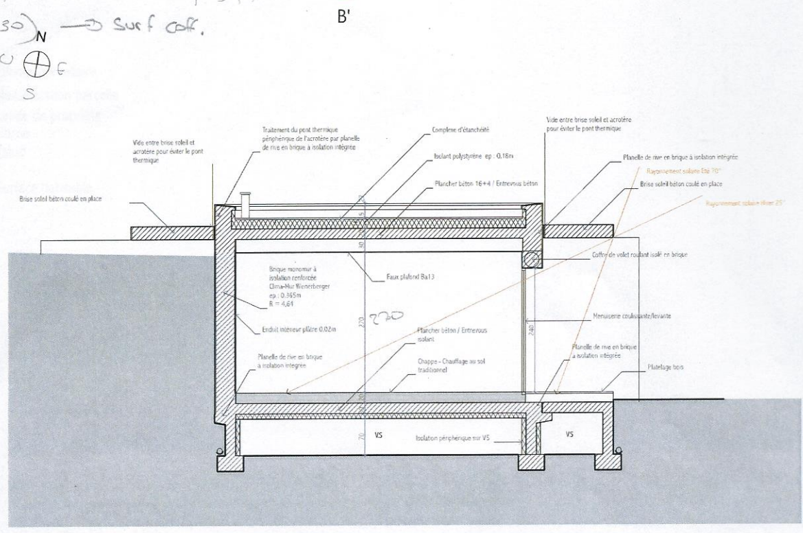
Coupe BB'
